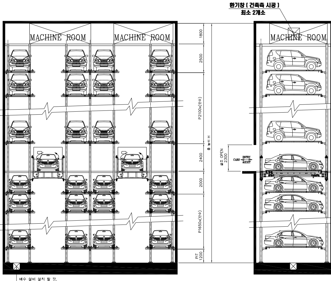
기계식주차장 정면도
