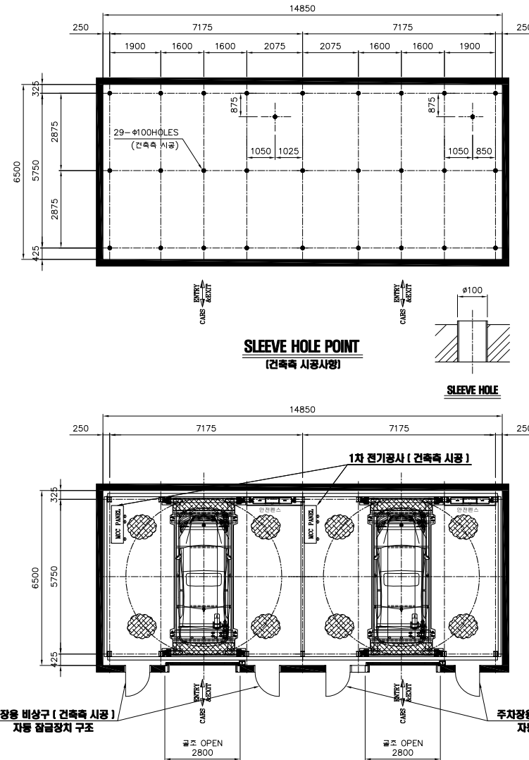
입고층 평면도
