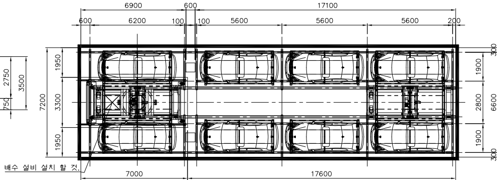
기계식주차장 평면도
