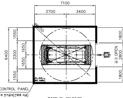
입고층 평면도
