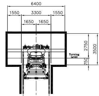
입고층 정면도 [180°]
