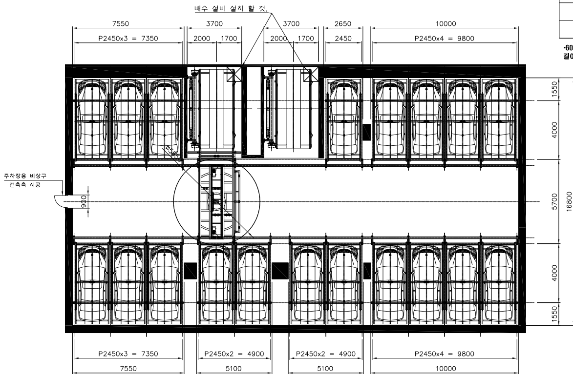
기계식주차장 평면도
