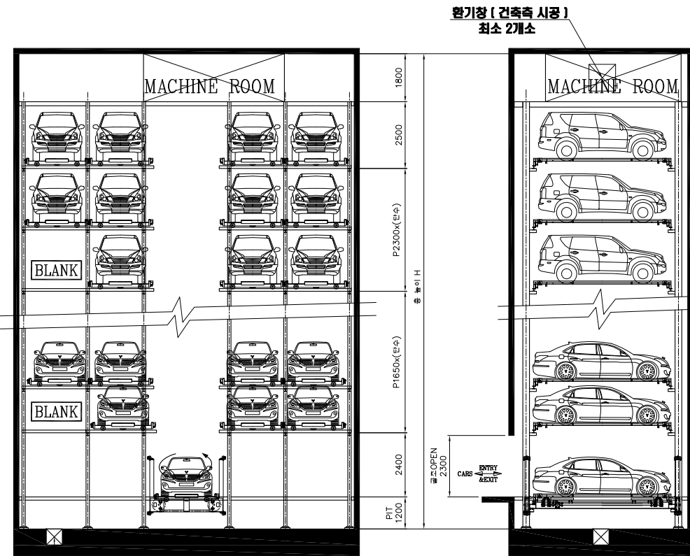
기계식주차장 정면도
