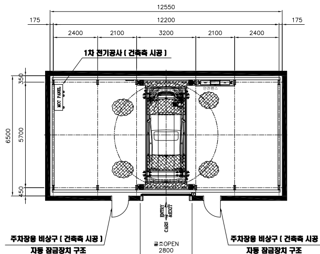
입고층 평면도
