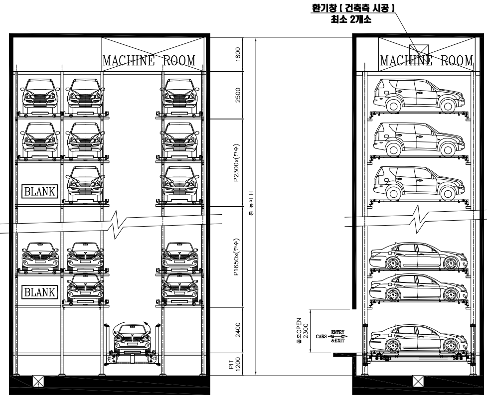
기계식주차장 정면도
