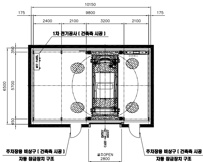
입고층 평면도
