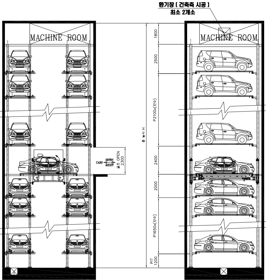
기계식주차장 정면도
