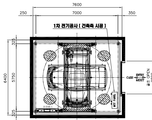
입고층 평면도
