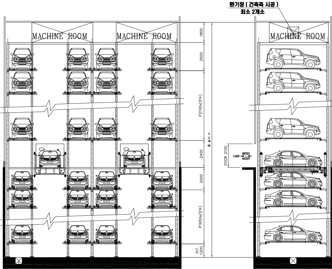
기계식주차장 정면도
