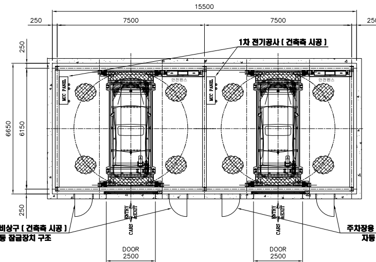
입고층 평면도
