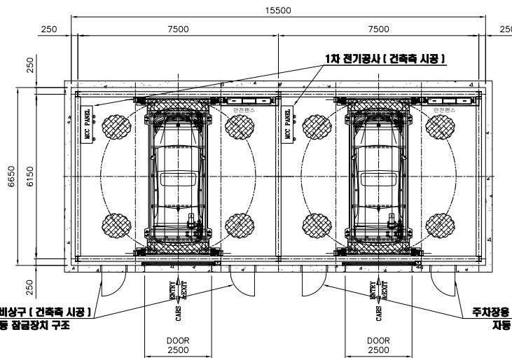
입고층 평면도
