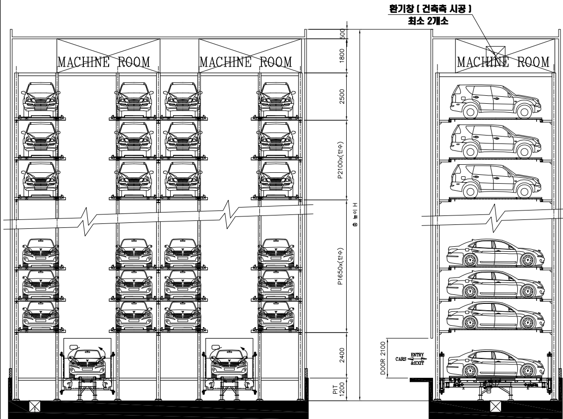
기계식주차장 정면도
