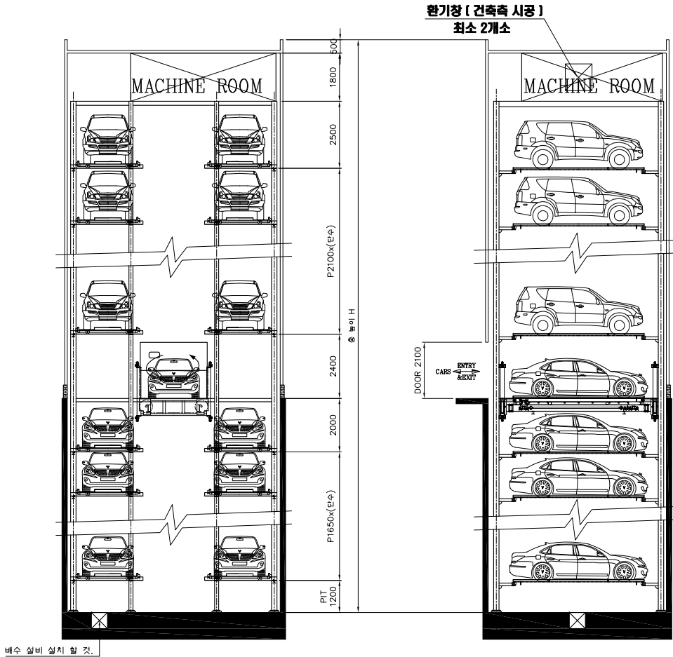
기계식주차장 정면도
