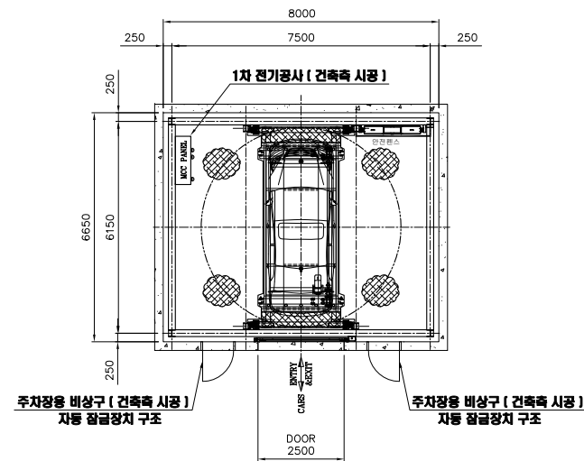
입고층 평면도
