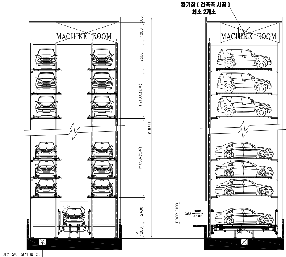
기계식주차장 정면도
