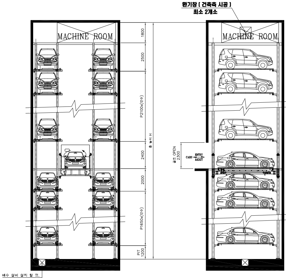
기계식주차장 정면도
